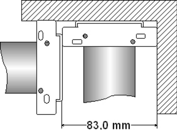
Systeem 45mm plaatsing: In de dag bovenaanzicht
